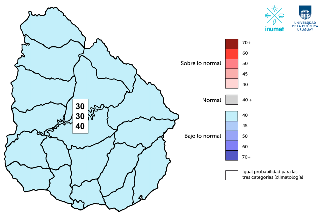
FIGURA 7 Probabilidades en porcentajes de los terciles de temperatura. Meses: octubre – noviembre – diciembre de 2026.
